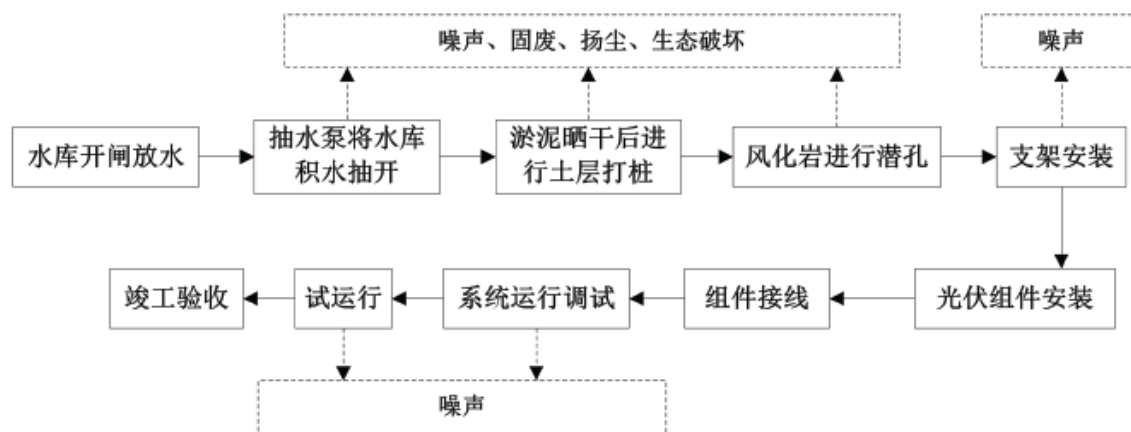
图 4-1 光伏区施工工艺流程及产污环节示意图
