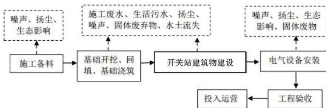
图 4-2 开关站施工工艺及产污环节示意图
